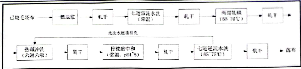
退浆丝光工艺流程图
