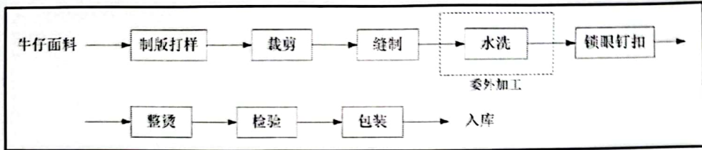
牛仔服装生产工艺流程图
